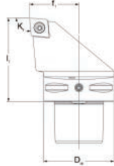
SCLCR/L-Kr 95°
