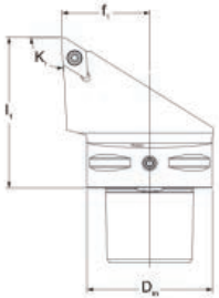
SDJCR/L-Kr 93°
