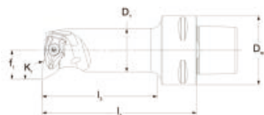
DDUNR/L-Kr93°
