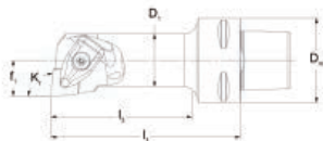
DCLNR L-Kr 95°
