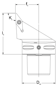
SVJBR/L-Kr 93°
