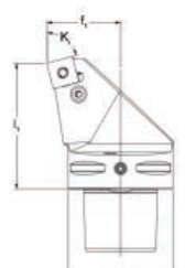
PSKNR/L-Kr 75°
